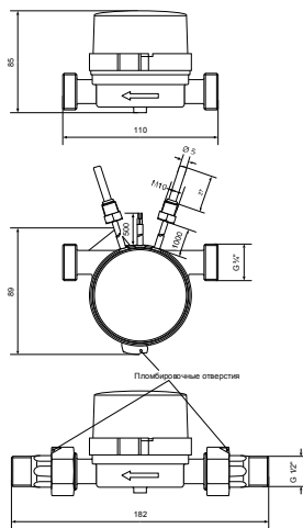
Рисунок 3. Счетчик тепла «Гефест xx.A2»
