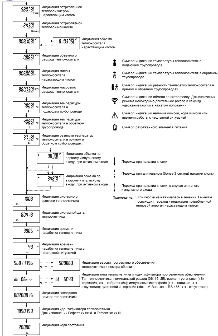
Рисунок 6. Последовательность переключения параметров на индикаторе теплосчетчика.
