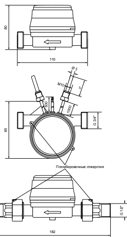
Рисунок 2. Счетчик тепла «Гефест xx.A1»
