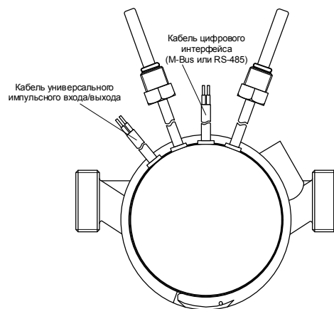
Рисунок 5. Расположение кабелей, проводных интерфейсов счетчиков тепла «Гефест», исполнений Гефест xx.IM и Гефест xx.IR.
