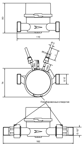
Рисунок 1. Счетчик тепла «Гефест xx.Vx»
