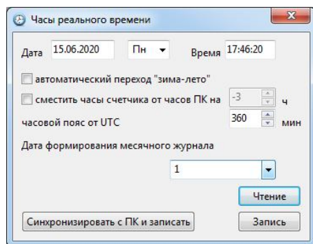
Рисунок 10. Окно «Часы реального времени»
