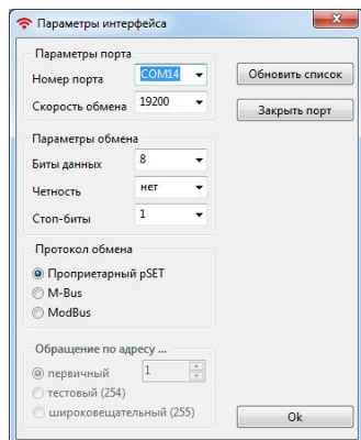
Рисунок 7. Окно «Параметры интерфейса»
